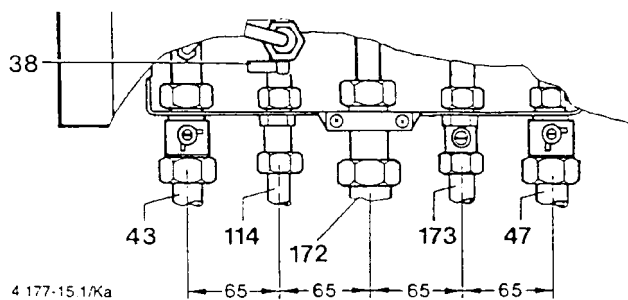
Figura 7 Montagem, placa de ligação, montada
