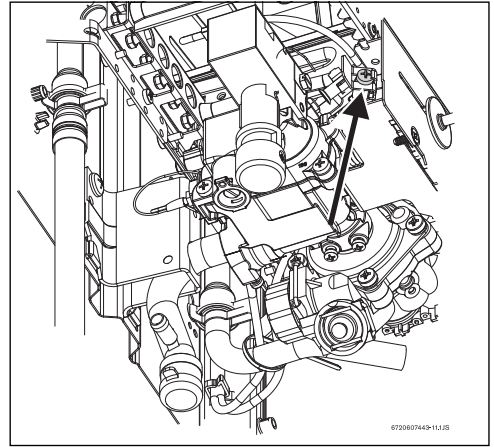
Fig. 14 Parafuso de ajuste de caudal de gás mínimo
