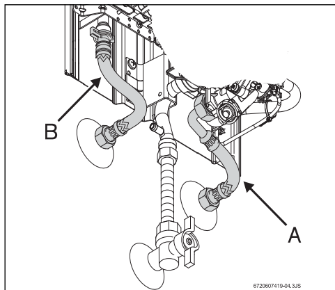
Fig. 11 Ligação da água
