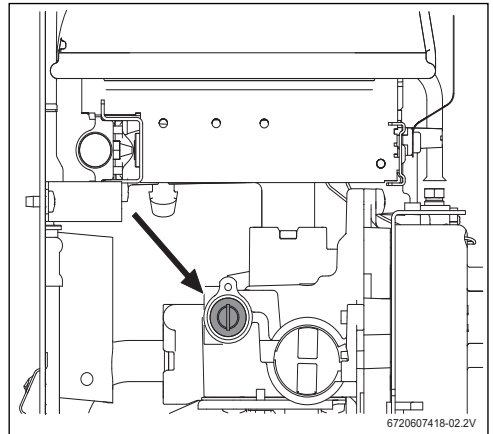
Fig. 15 Parafuso de ajuste de caudal de gás máximo
