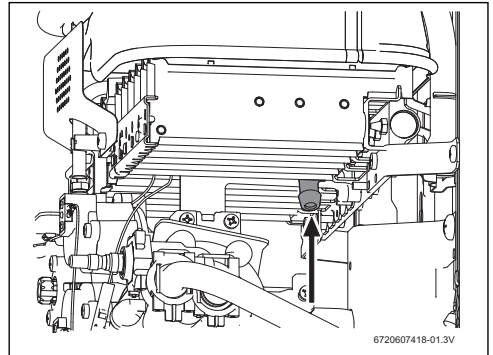
Fig. 14 Ponto de medição de pressão
