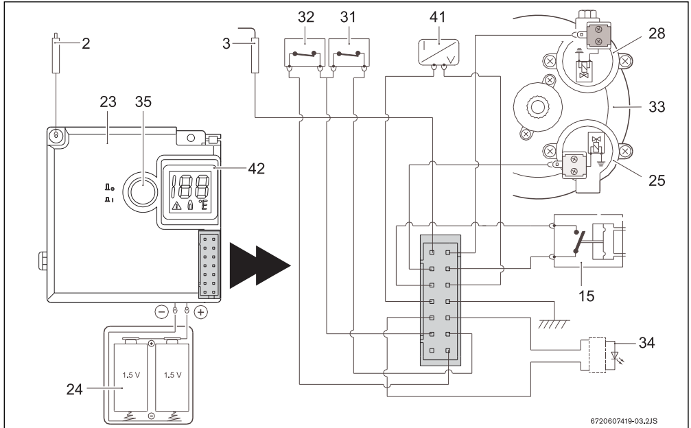
Fig. 2 Esquema eléctrico
