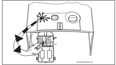
Fig. 5 Substituição das pilhas
